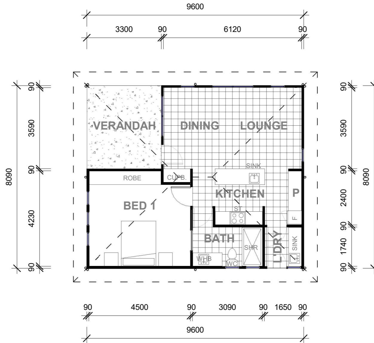
1 FLOOR PLAN 1 : 100
