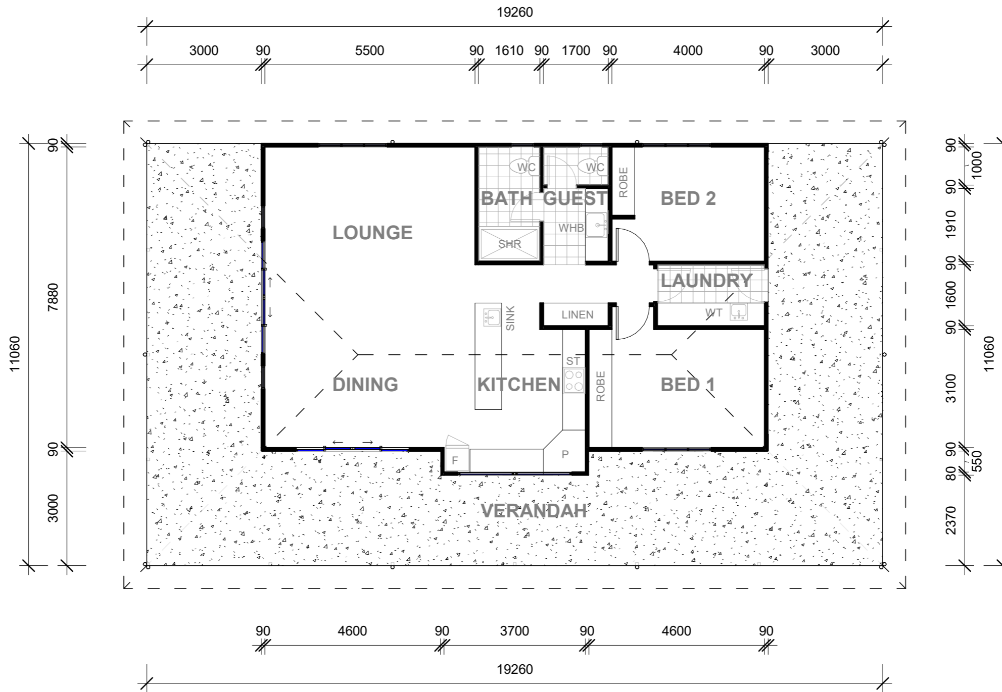
1 FLOOR PLAN 1 : 100
